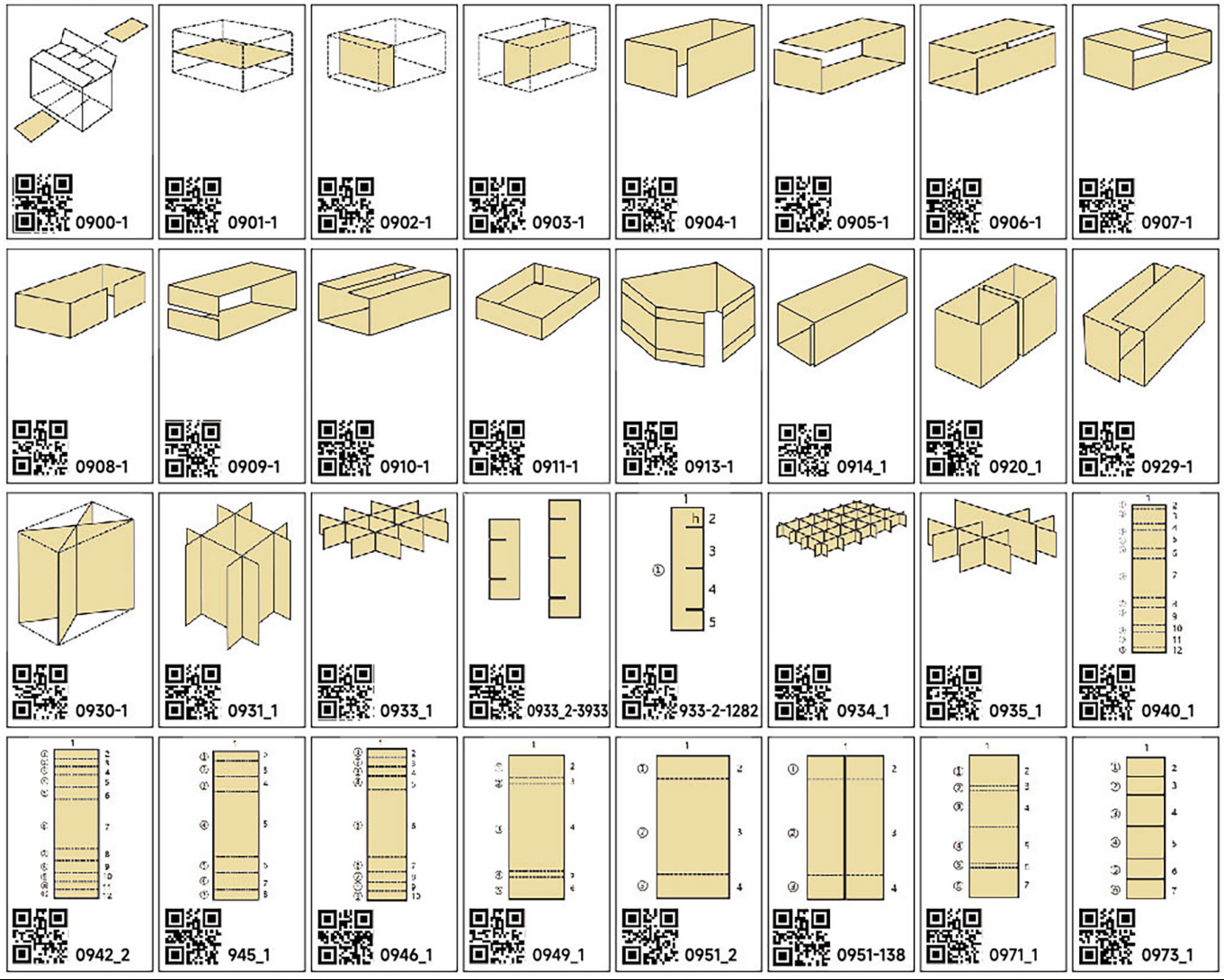
0900 系列盒型
